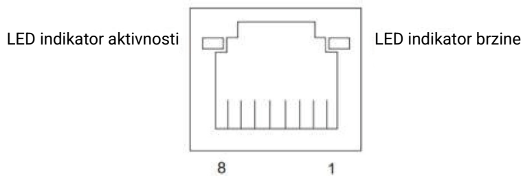
Slika 13. Priključak RJ45 (strana na kojoj je priključak)
