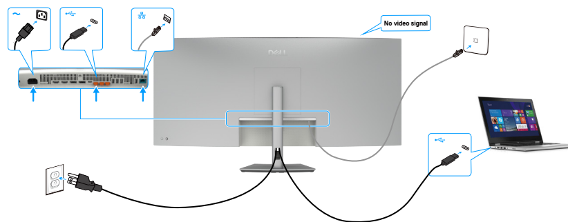
Slika 33. Mrežno usmeravanje preko USB-C dolaznog priključka
