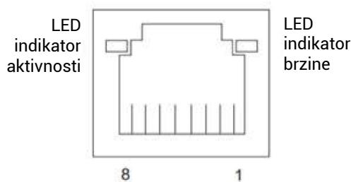
Slika 10. Priključak RJ45 (strana na kojoj je priključak)
