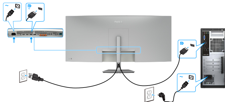
Slika 29. Priključivanje DisplayPort kabela
