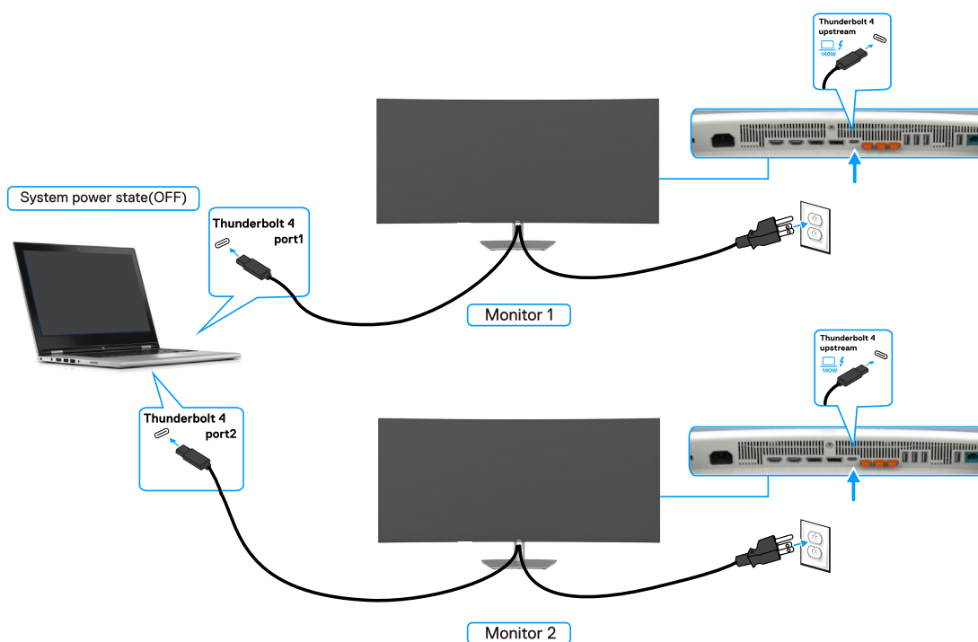
Slika 49. Stanje napajanja dva monitora i računara Isključeno u DPBS režimu
