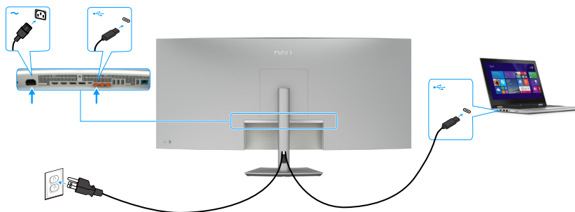
Slika 32. Priključivanje USB-C kablova (C na C) (opciono)
