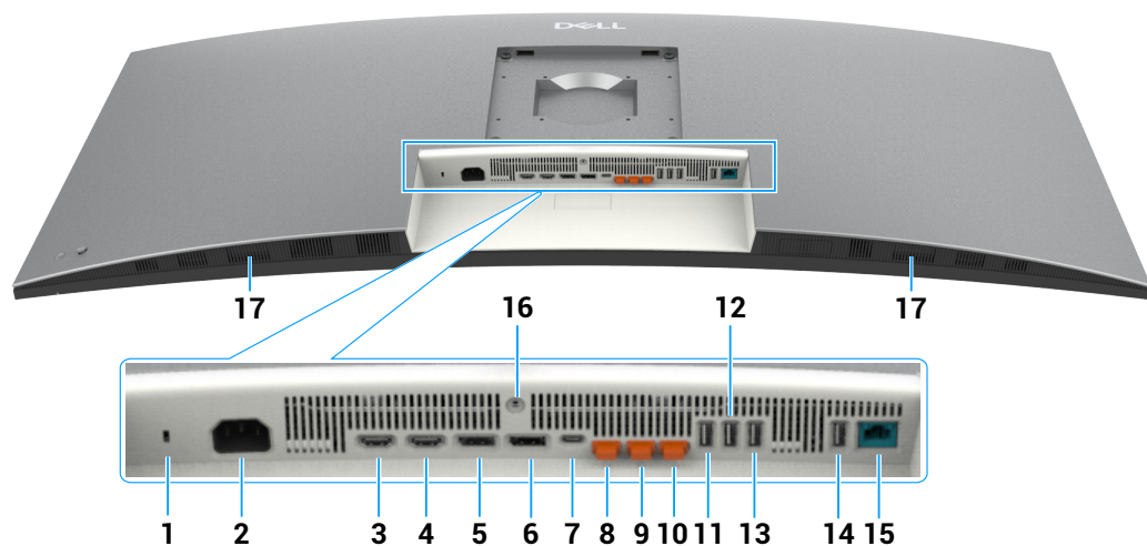
Slika 4. Pogled odozdo
